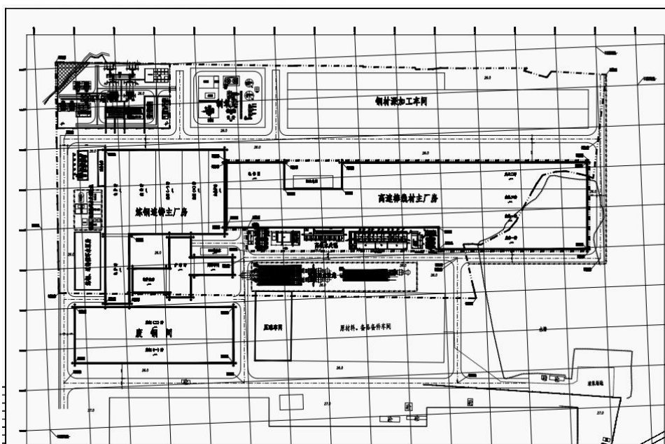
图 3-2 企业厂区平面布置图
